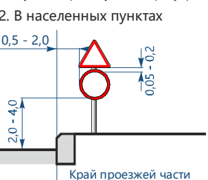
Размещение знаков на опоре
